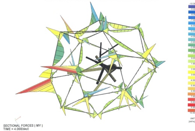
12) Vent selon - X- Etat de dimensionnement (TIME 4) – tube 101.6 toiture seulement Moments de flexion MY « vue de dessus »
